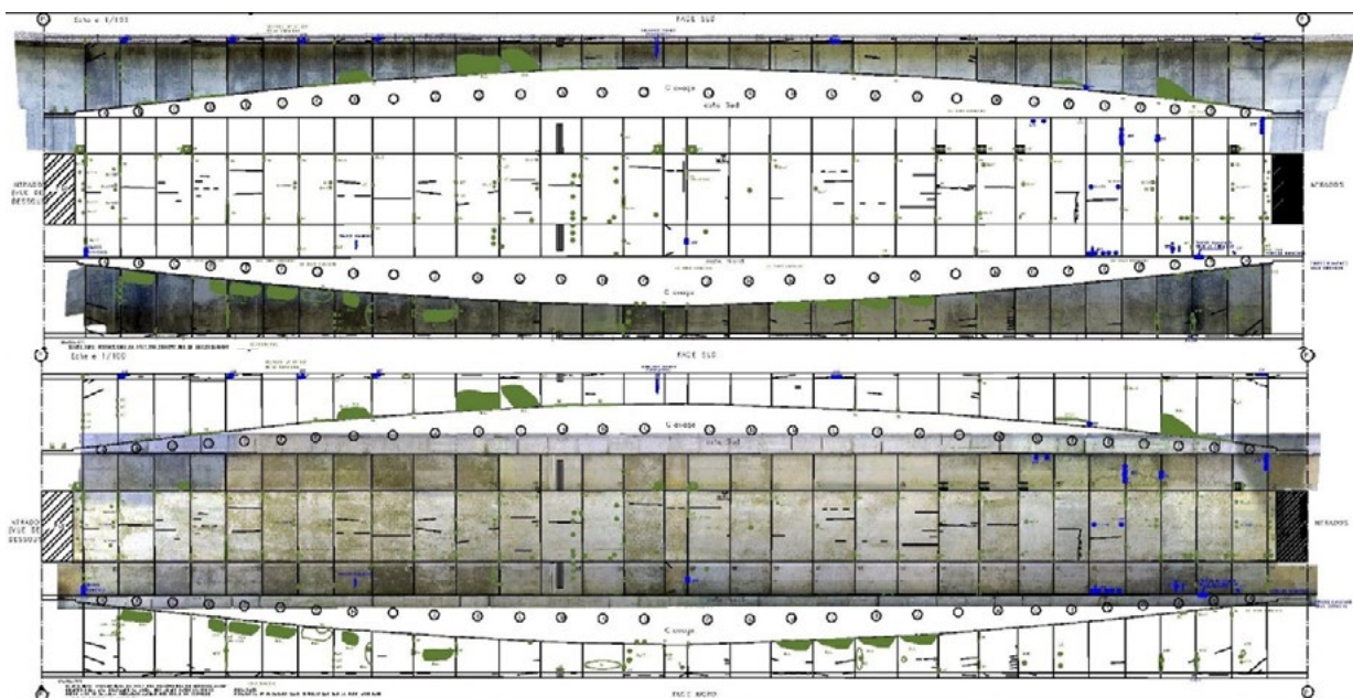
► Figure 36 : Relevé de désordre sur orthophotographie
