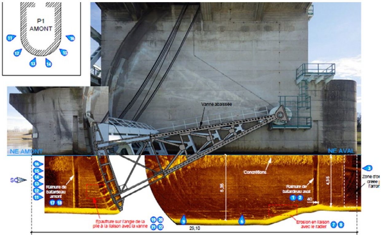
► Figure 37 : Relevé de désordre sur une partie immergée d'un barrage
