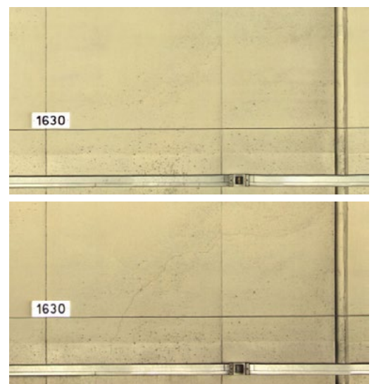
► Figure 20 : Comparaison entre deux inspections, apparition d'une fissure sur piedroit de tunnel à 3 ans d'intervalle
