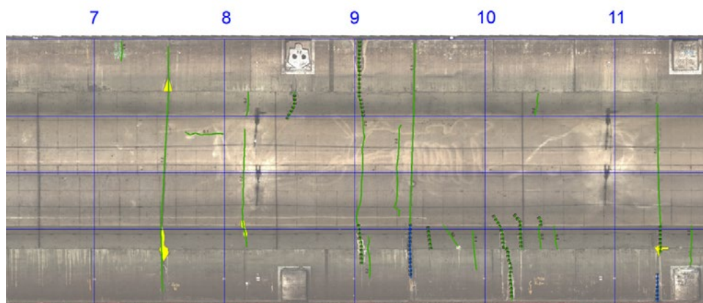
► Figure 40 : Relevé de désordres sur une orthophotographie générée à partir du modèle 3D précédent
