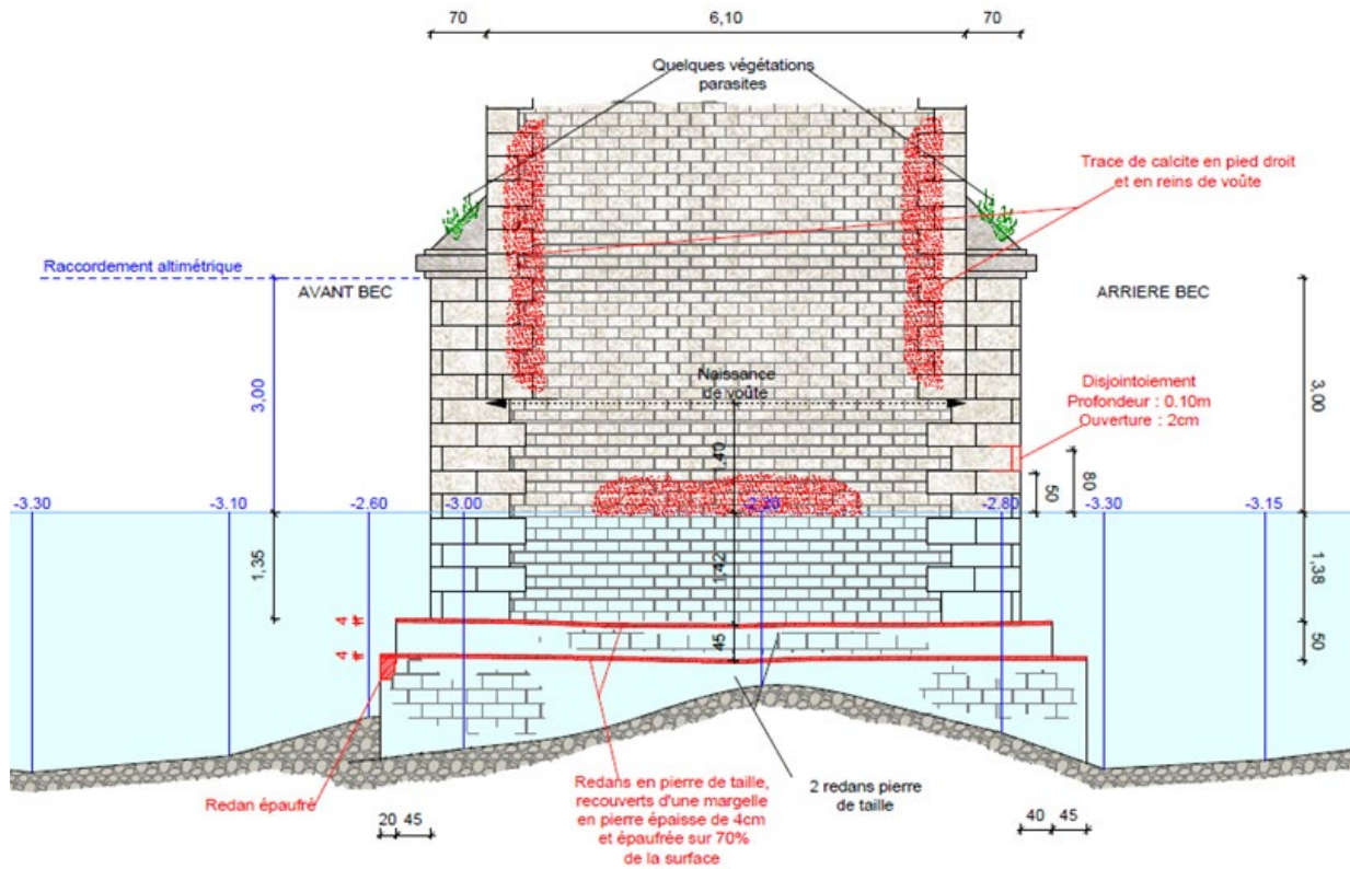
► Figure 26 : Vue en élévation d'une pile avec représentation des désordres
