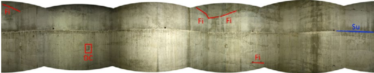
► Figure 24 : Mosaïque à 360° de l'intérieur d'une pile de pont
