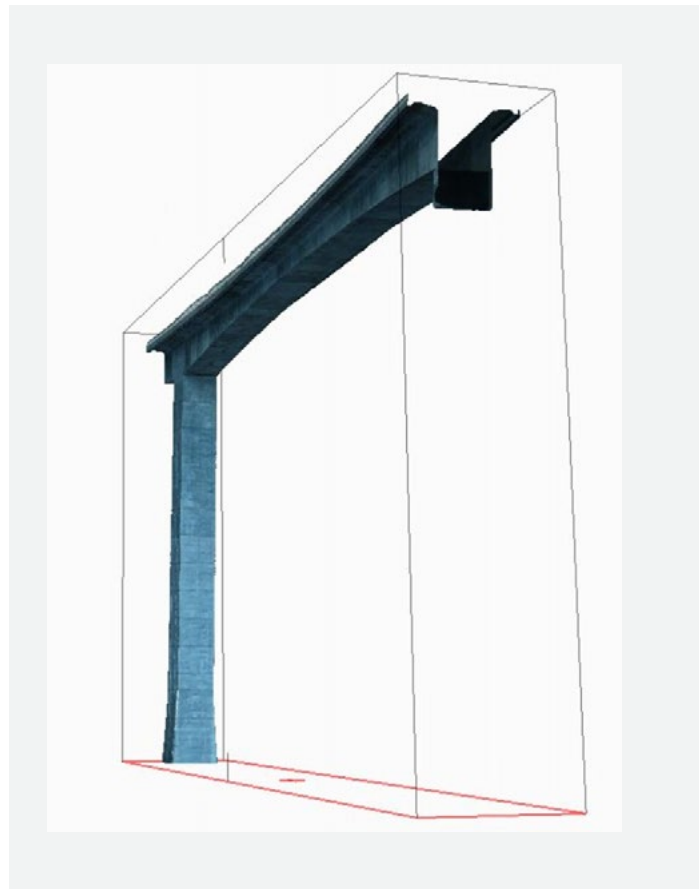
► Figure 17 : Modèle 3D issu de la reconstitution par photogrammétrie d'un viaduc
