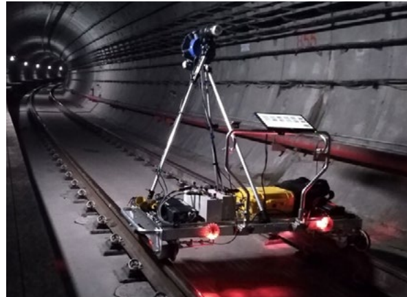
► Figure 4 : Système d'acquisition de photo-profil en tunnel
