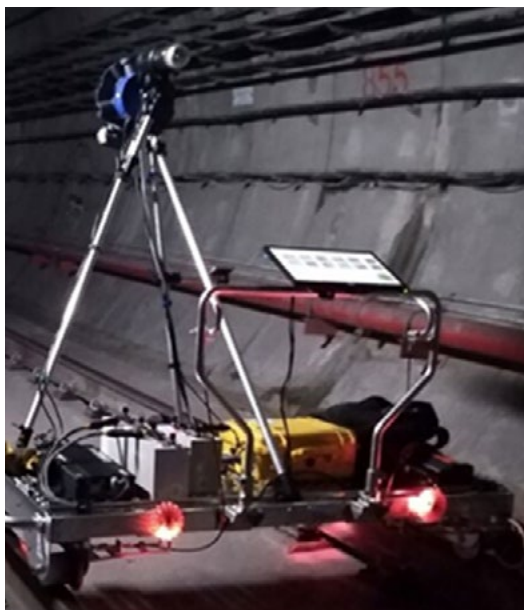
► Figure 38 : Système d'acquisition par photo-profils
